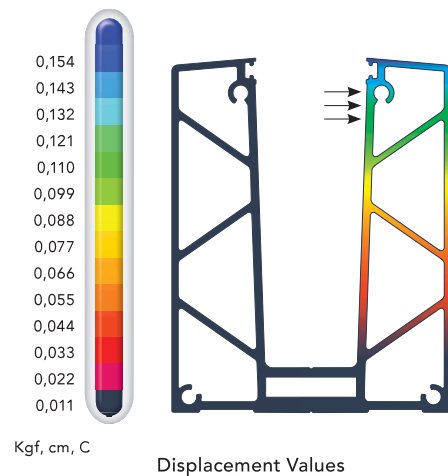
Displacement Values
